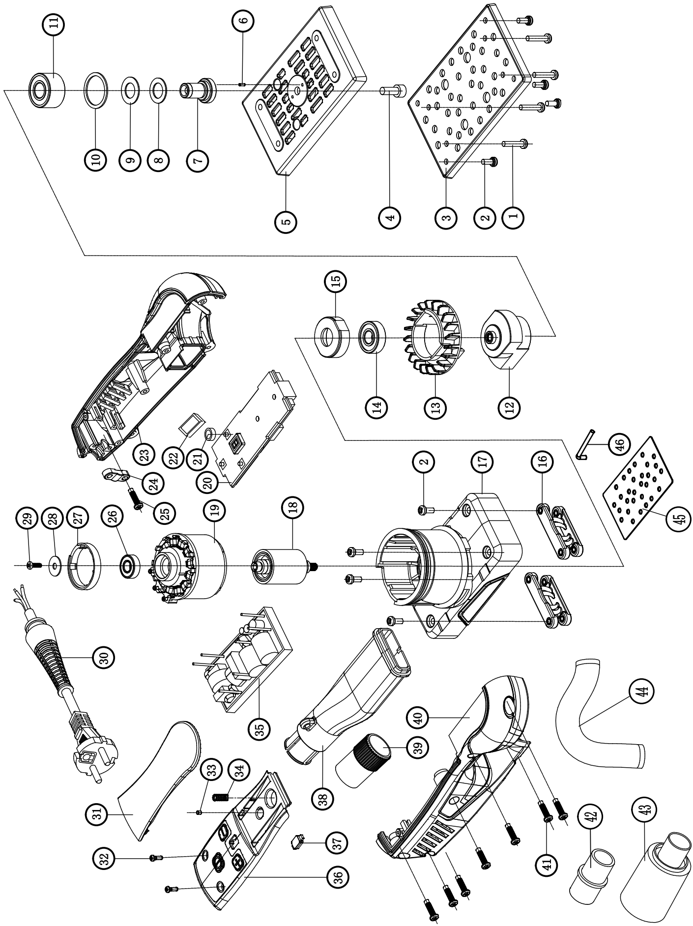
S1B-HD02-80×133爆炸图
